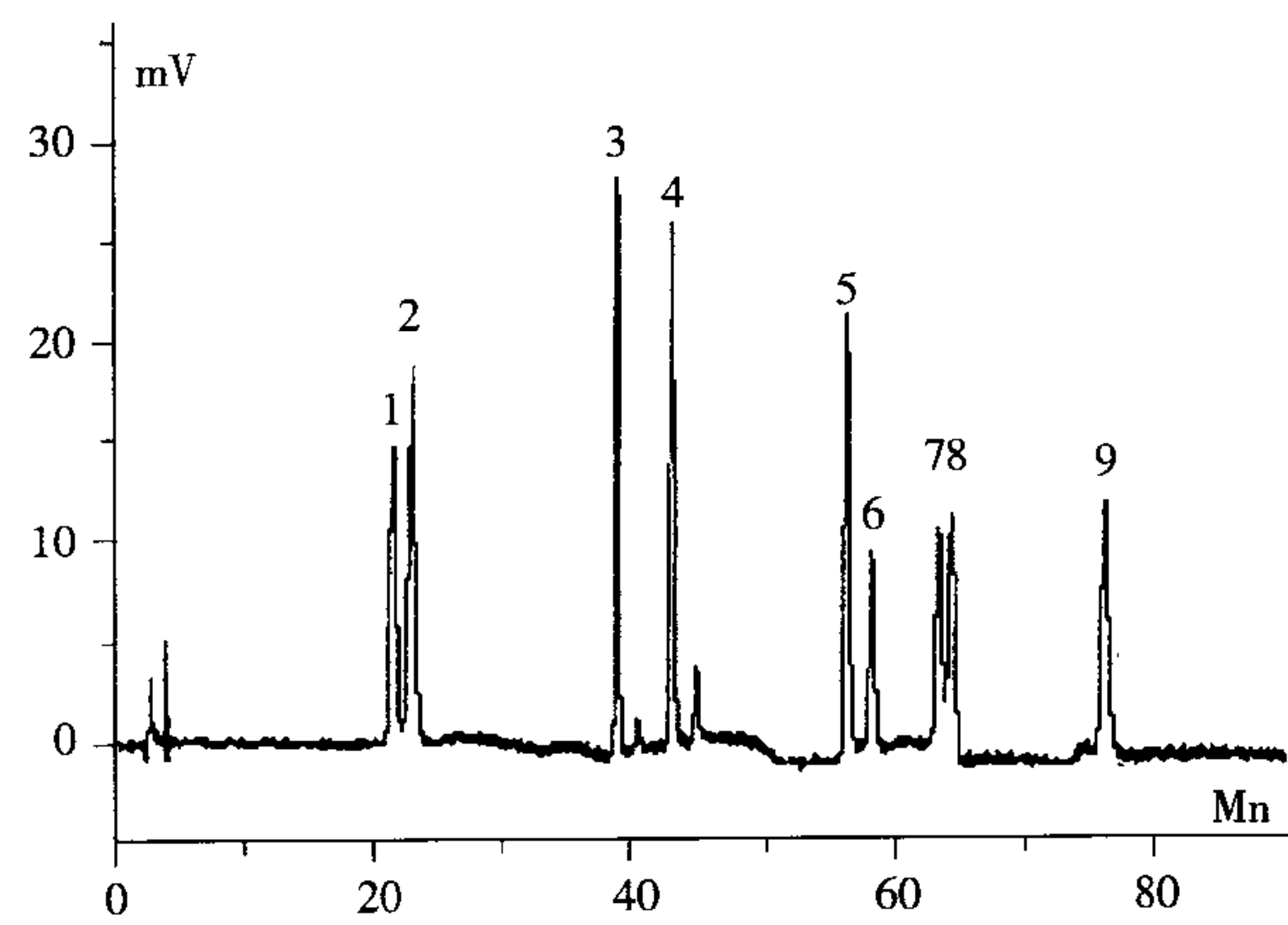
图 A. 1 9 种人参皂苷标准品的液相色谱图
